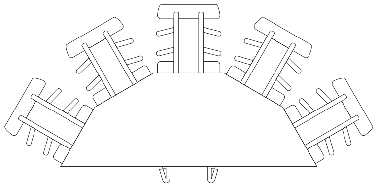
SWIGGLE STARBURST 5.5 x 18 5 POS. WHT - BI 292001 ALM - BI 292054 CL - BI 292051
